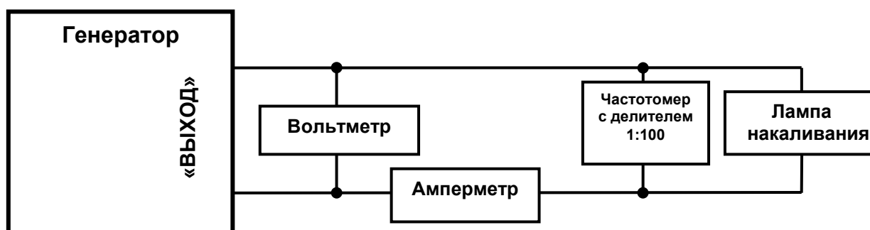
Рисунок 7.5.2 – Схема рабочего места для проверки параметров генератора
