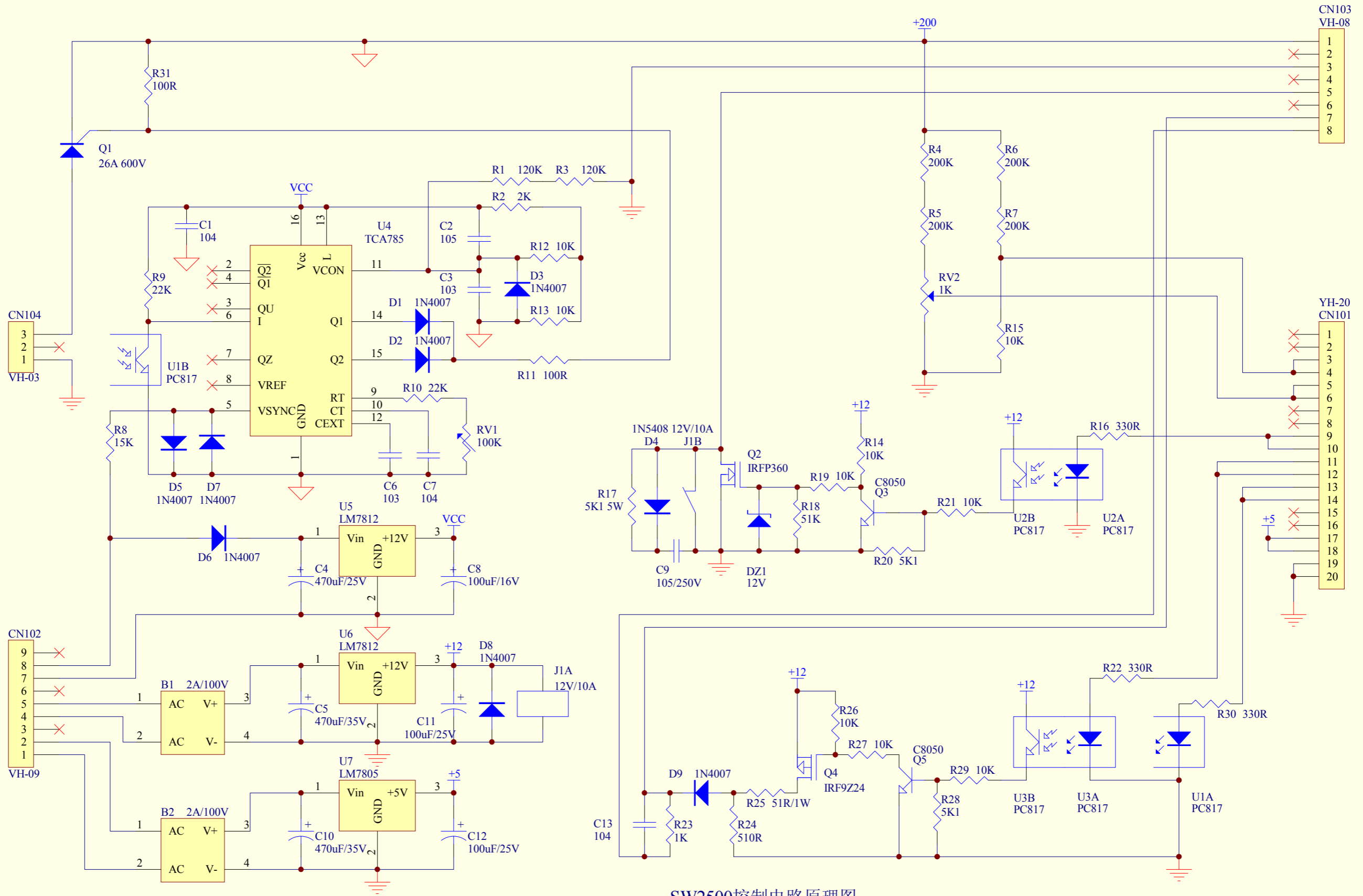
SW2500控制电路原理图
