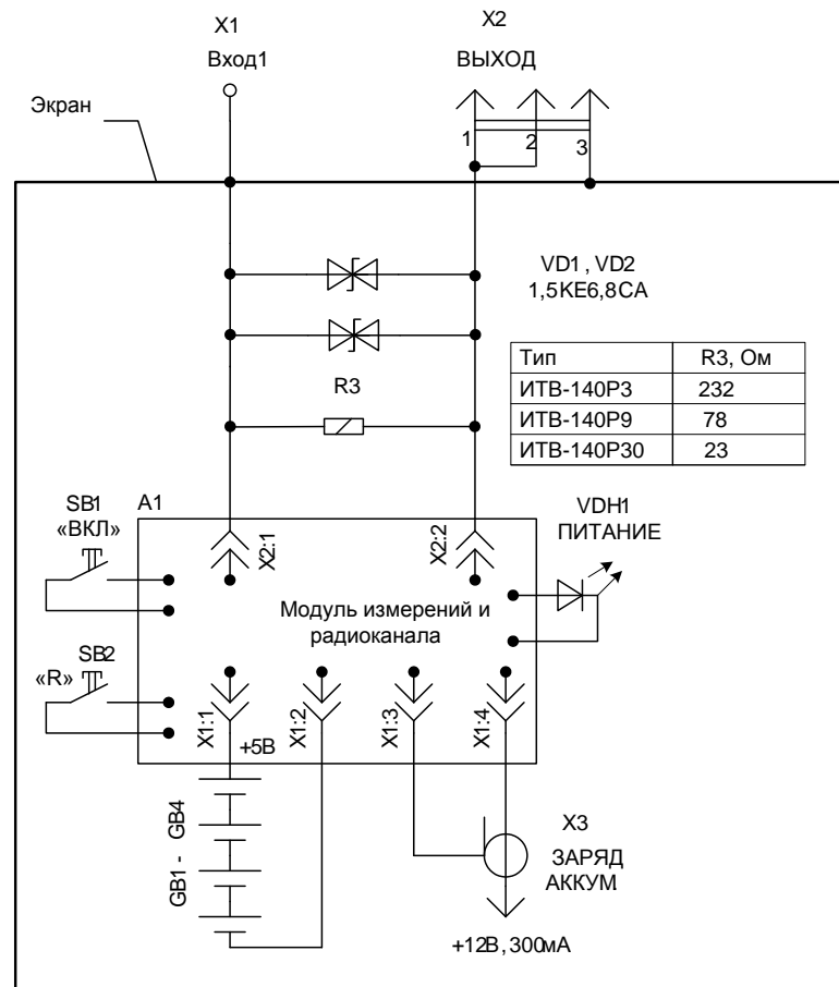
Рисунок 1. Блок высокопотенциальный ИТВ-140Р-БВ. Схема электрическая принципиальная.
