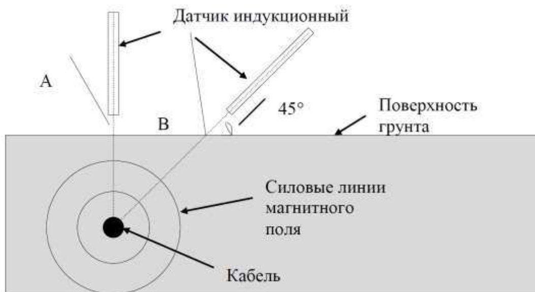
Рисунок 17. Определение глубины залегания кабеля.
