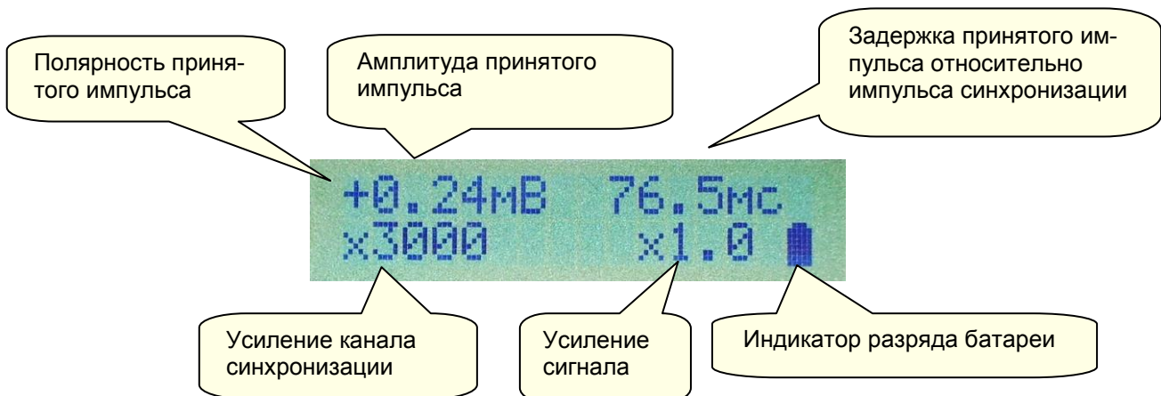
Рисунок 4. Режим акустического датчика
