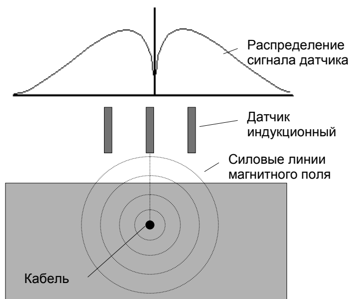
Рисунок 6. Поле кабеля в режиме трассы при вертикальном положении индукционного датчика
